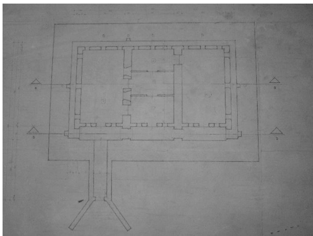
Plattegrond en vooraanzicht kazemat op bastion VIII.
